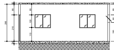
CORTE BB ESCALA 1/50
