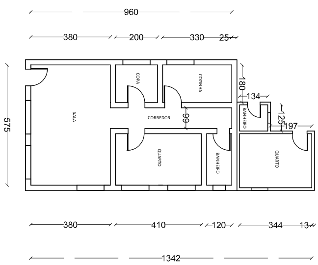
PLANTA BAIXA BL 03 ÁREA = 75,84 M 2 ESC: 1:50
