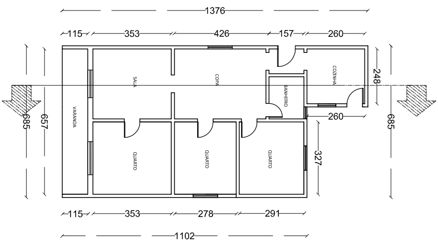
PLANTA BAIXA BL 01 ÁREA = 82,64 M 2 ESC: 1:50
