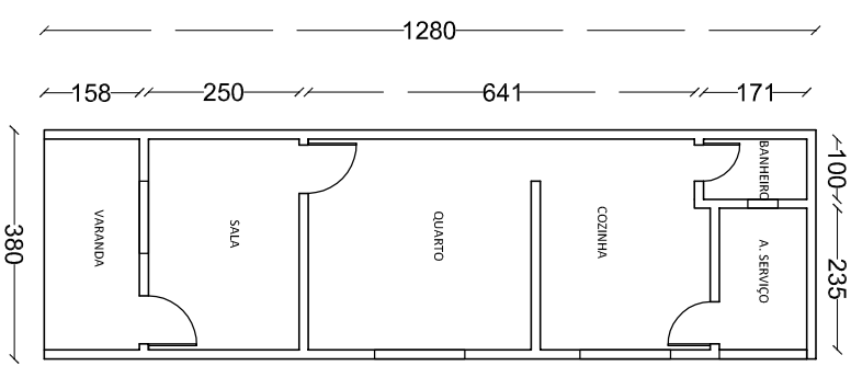
PLANTA BAIXA BL 02 ÁREA = 48,64 M 2 ESC: 1:50
