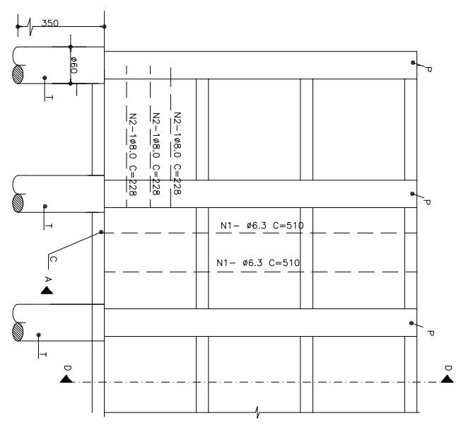
ELEVACÃO DETALHE DA ARMAÇÃO ESC. 1:50
