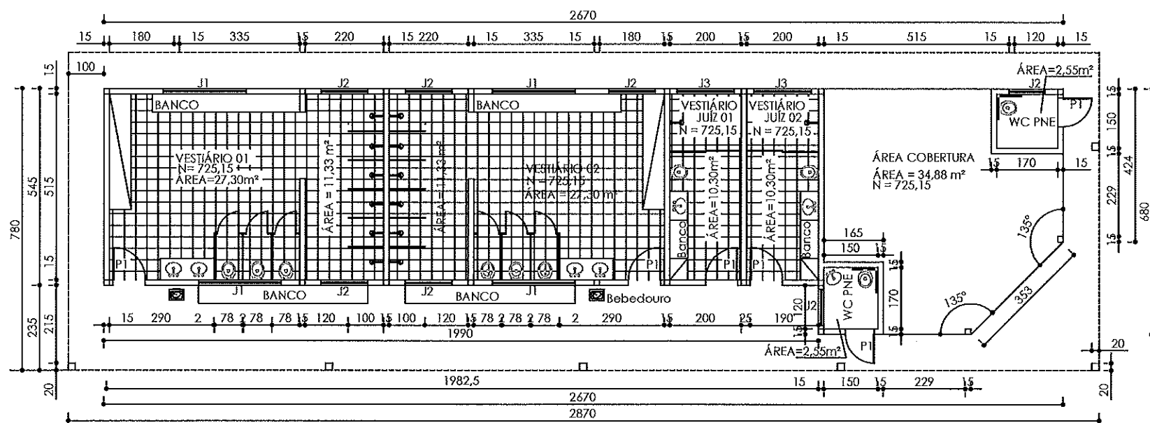
PLANTA VESTIÁRIO - CAMPO DE ROÇA GRANDE ESCALA 1:100
