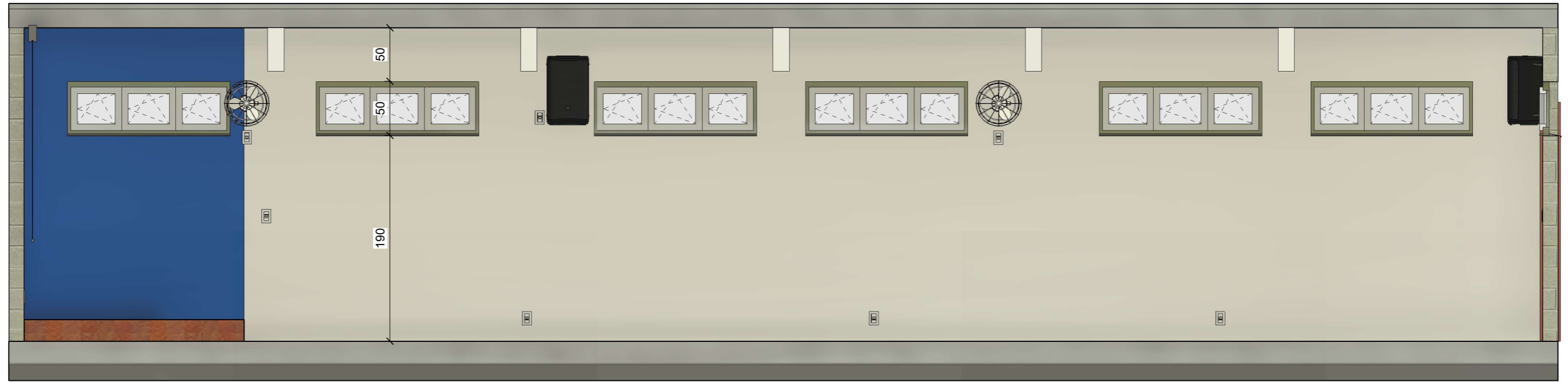
1 Corte DD 1 : 20
