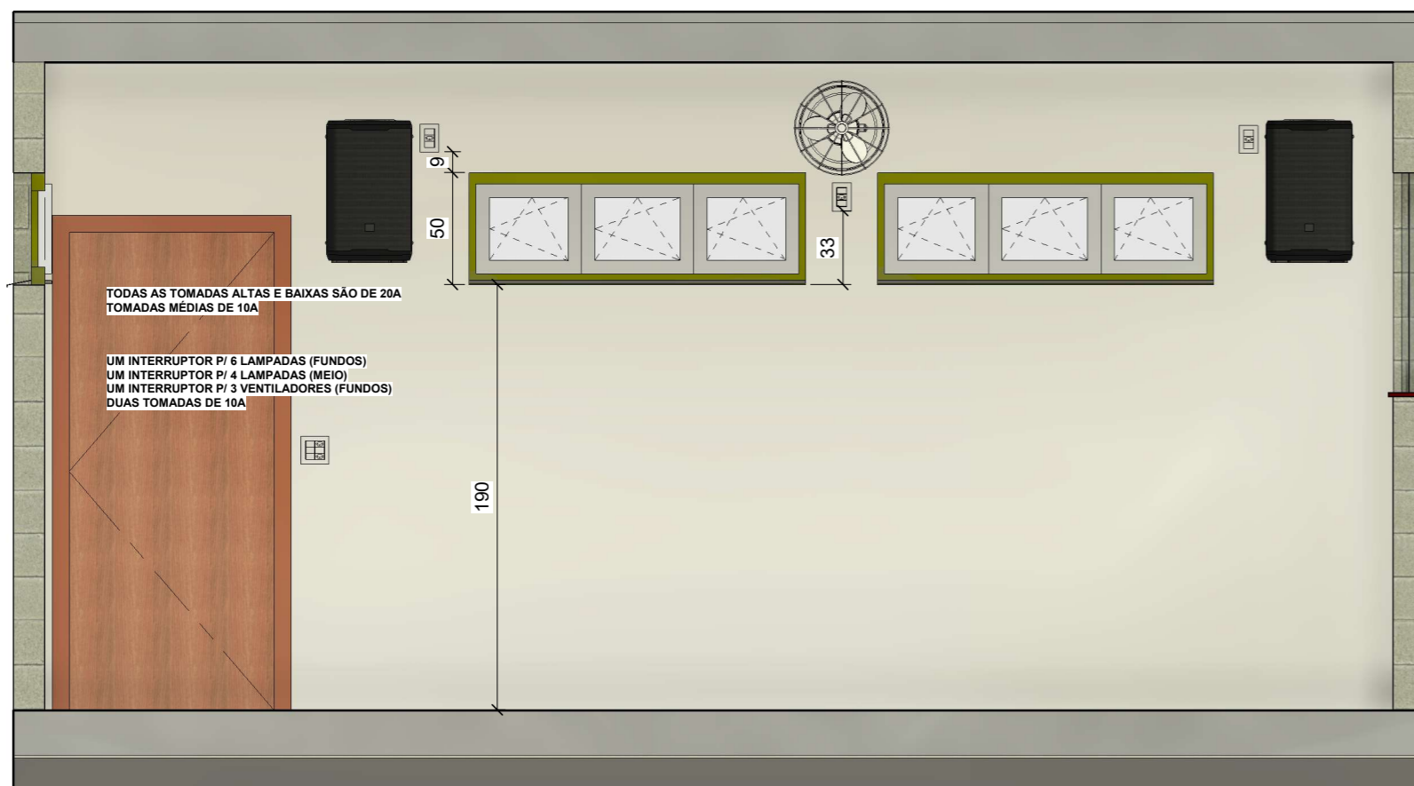
1 Corte BB 1 : 15
