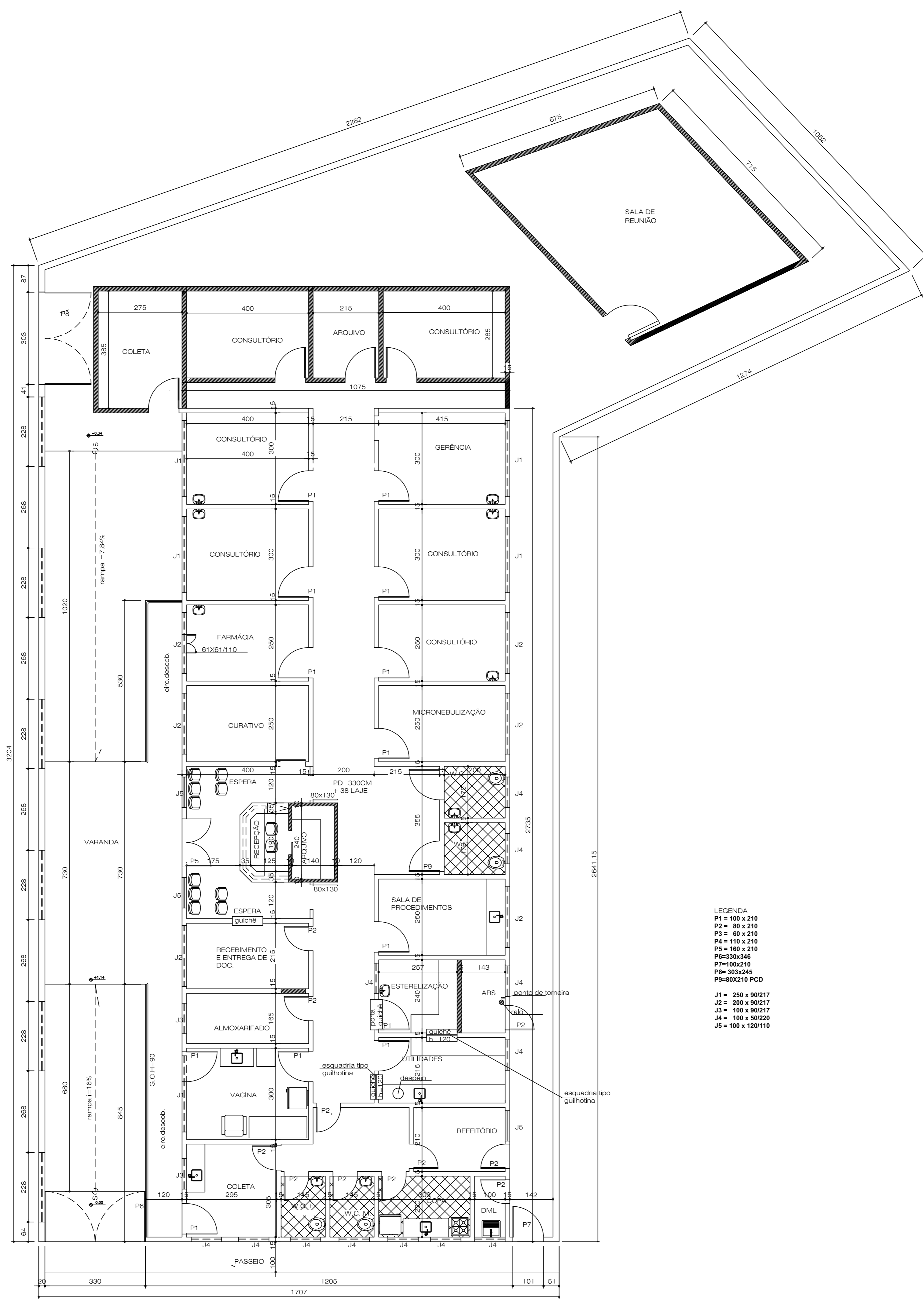
PLANTA PAVTO TÉRREO ESCALA: 1/75 ALVENARIA A CONSTRUIR
