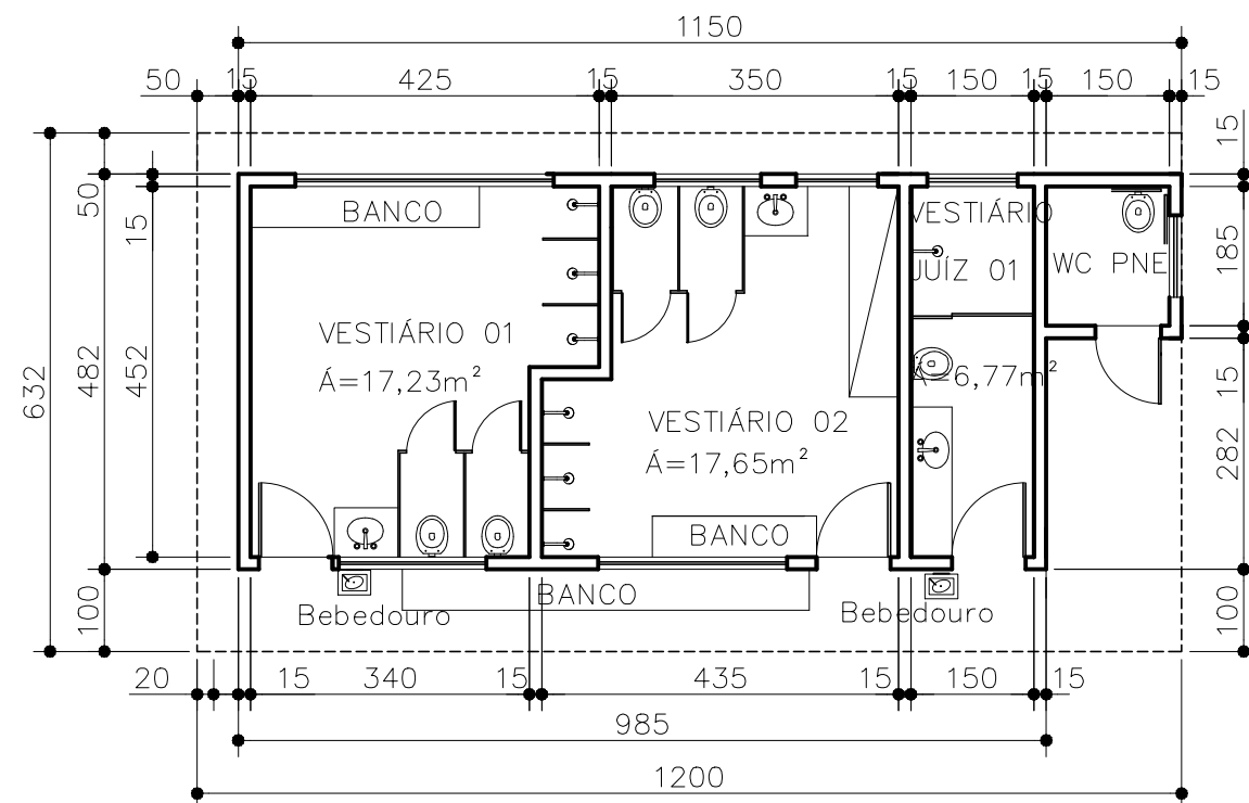
PLANTA VESTIÁRIO – CAMPO CUTAPA ESCALA 1:100
