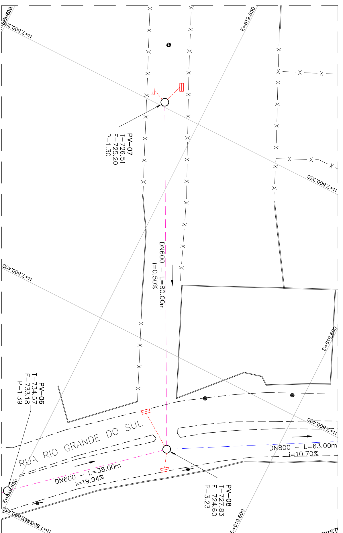
PLANTA – RUA SEM NOME E RUA RIO GRANDE DO SUL ESC. 1:500
