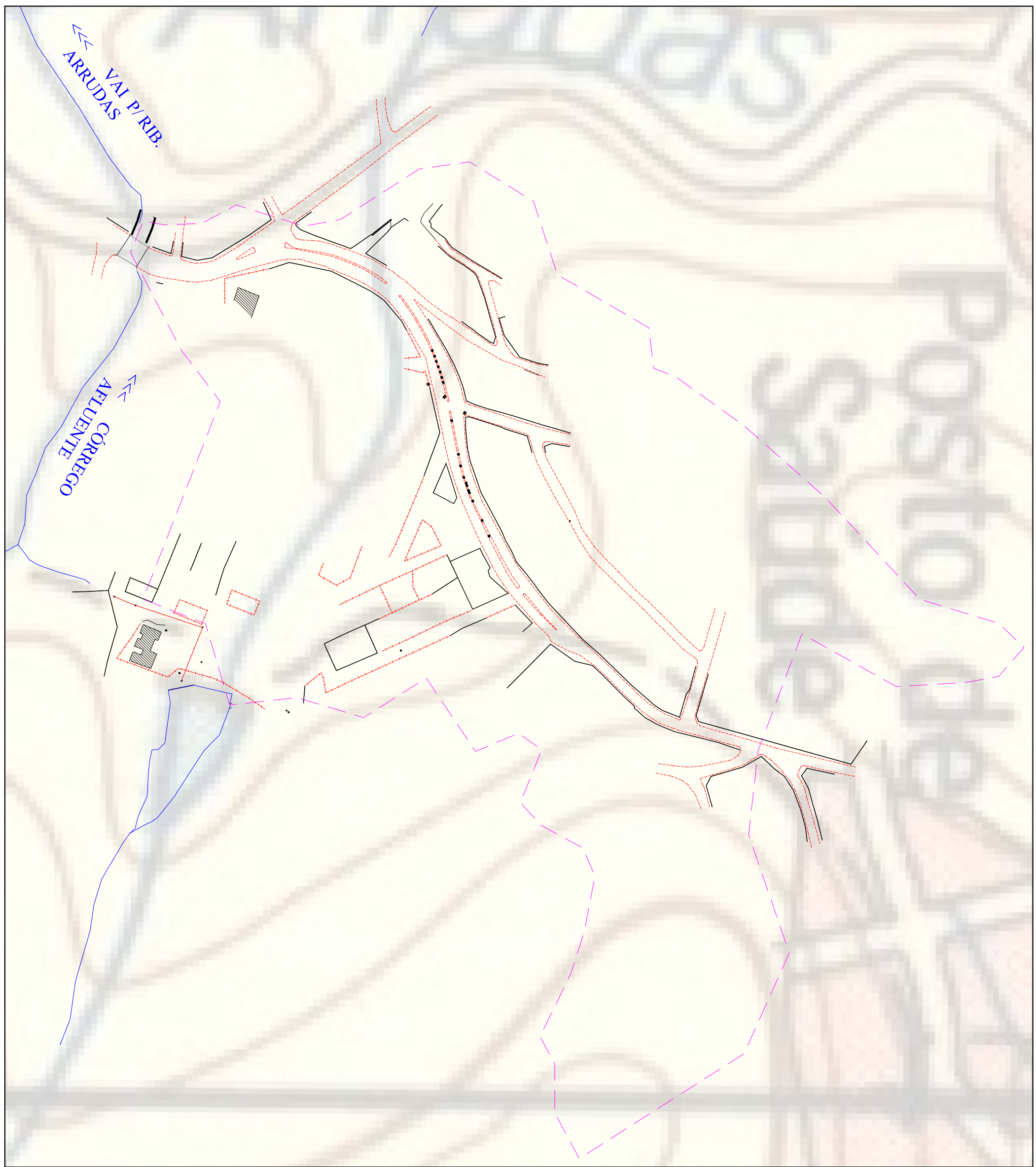
DEFINIÇÃO DOS LIMITES DA BACIA DE DRENAGEM COM AUXÍLIO DE CARTOGRAFIA EXTRAÍDA DA BASE DE DADOS DO IBGE Esc. 1:2.500
