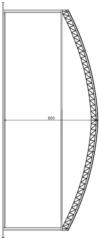
CORTE J-J ESC. 1/50
